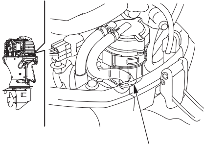
ВЛАГООТДЕЛИТЕЛЬ
