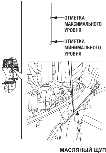
МАСЛЯНЫЙ ЩУП
