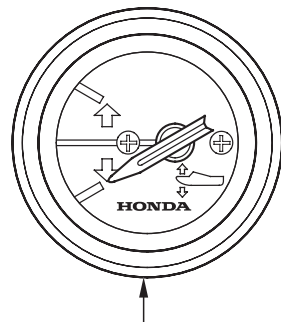
УКАЗАТЕЛЬ УГЛА ДИФФЕРЕНТА
