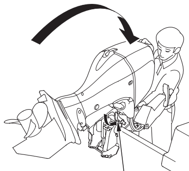
РЫЧАГ ФИКСАТОРА МОТОРА В ПОДНЯТОМ СОСТОЯНИИ
