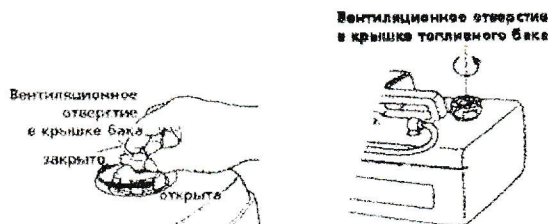
Вентиляционное отверстие в крышке топливного бака
