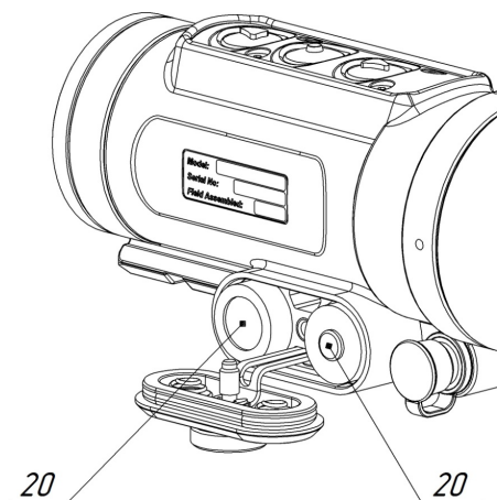
Рис.30 – Установка элементов питания
