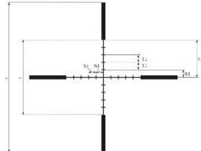
Рисунок 40 – Прицельная сетка (размер в м/100м дистанции)
