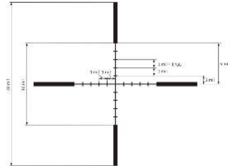
Рисунок 39 – Прицельная сетка (размер в миллирадианах или в т.д.)
