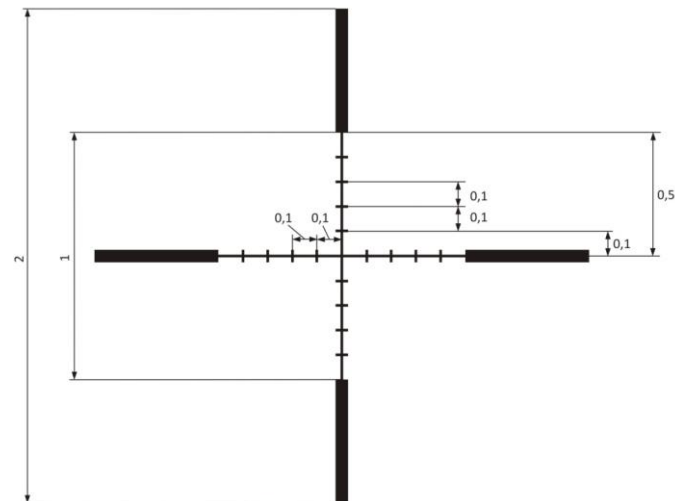
Рисунок 30 – Прицельная сетка (размер в м/100м дистанции)
